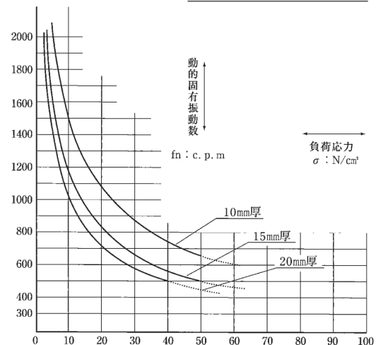
防振パット応力 - 固有振動数
